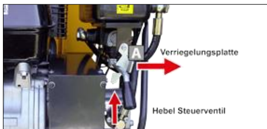
Hendelregelklep (6) voor het verhogen en verlagen van de kiepbak
