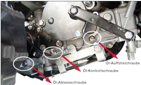
Versnellingsbakblok met olieregelpug, aftapplug en opblaasplug
