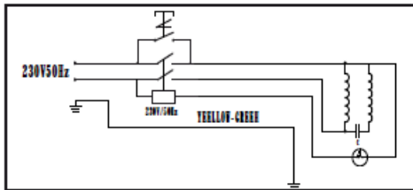
Schakelschema 230V-50Hz
